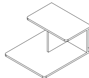
F10 L 600 x D 675 x H 300
