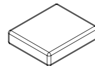
F1 (x1) L 600 x D 675 x H 150
