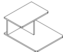
F10 (x1) L 600 x D 675 x H 300
