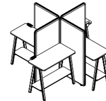
Screen (LxH) : 900 x 1650 mm | Table (LxWxH) : 1200 x 600 x 1050 mm
